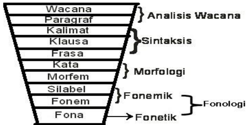
Gambar 1. Subsistem Bahasa
