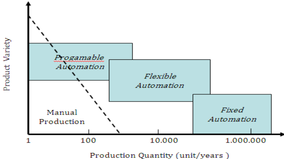
Gambar 2. Diagram P–Q Klasifikasi Otomasi (Sumber: Groover, hal.12, 2001)
